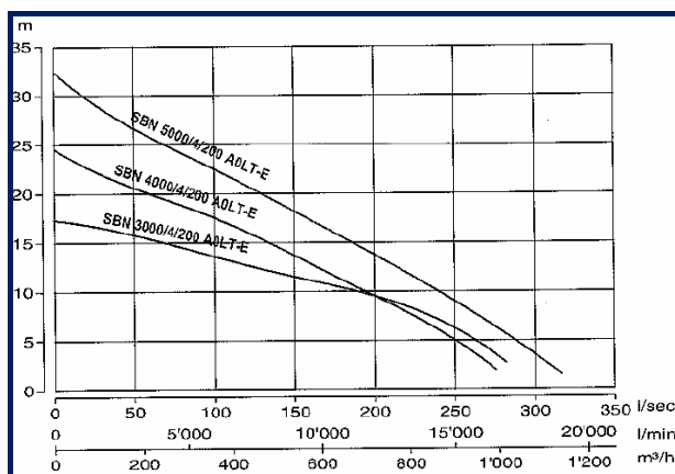
Diagramma 01 – Caratteristiche di funzionamento
