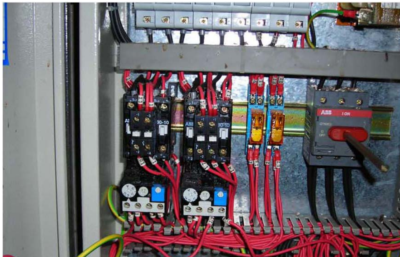
Fotografia 06 – Quadro elettrico
